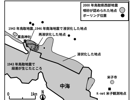
図-1 米子市における液状化地点
