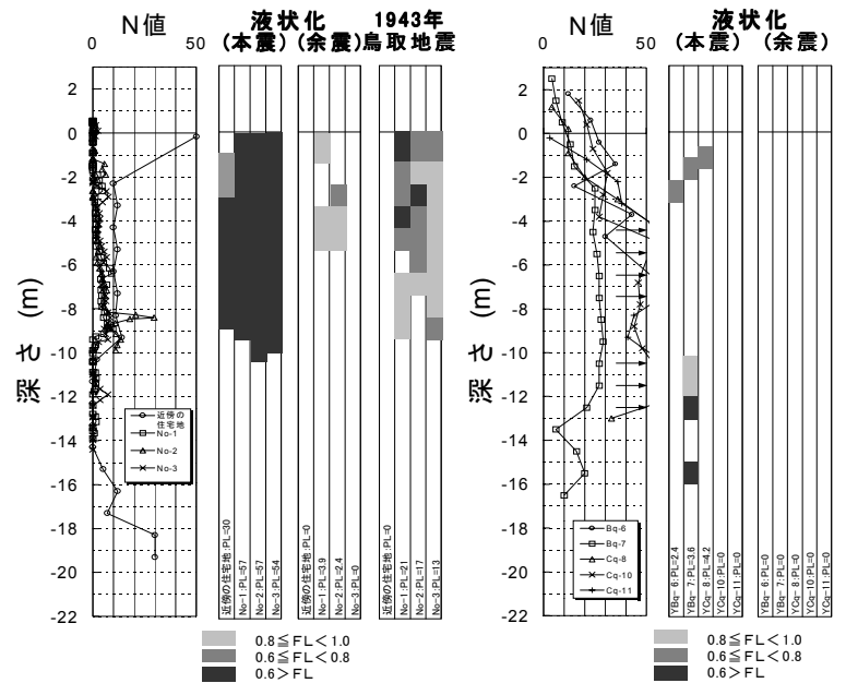
図-3 地盤柱状図と液状化判定
