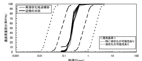
図-2 粒径加積曲線
