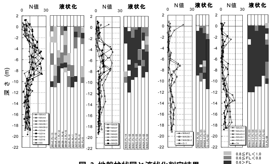
図-3 地盤柱状図と液状化判定結果
