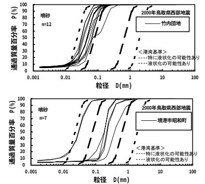
図-2 粒径加積曲線 (竹内団地,昭和町)
