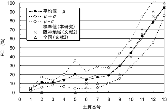
図1 土質ごとの細粒分含有率 FC
