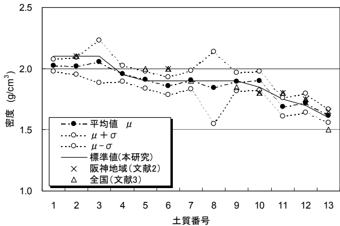
図3 土質ごとの密度 \rho_t
