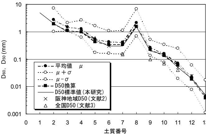
図2 土質ごとの60%粒径 D_{60} および平均粒径 D_{50}
