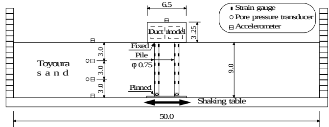
図-1 実験概要
