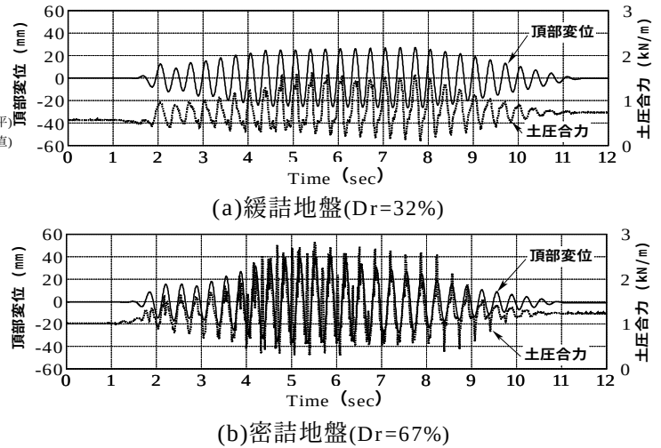
図-2 構造物頂部変位と土圧合力の時刻歴
