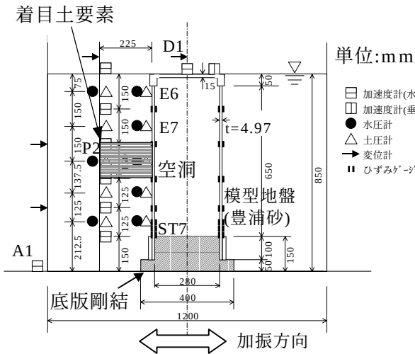
図-1 構造物模型および計測器配置
