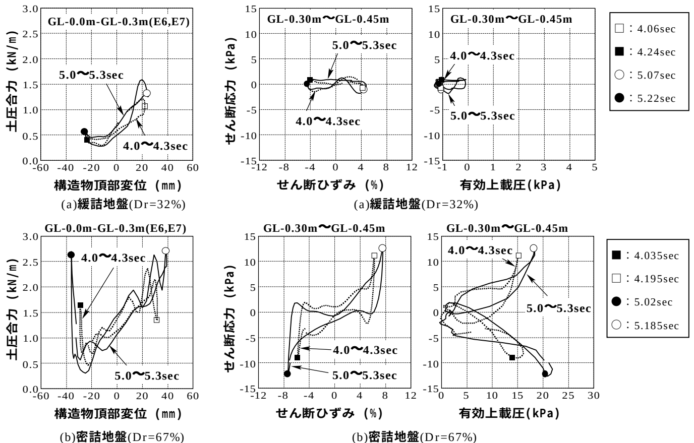
図-3 土圧合力と頂部変位の関係
