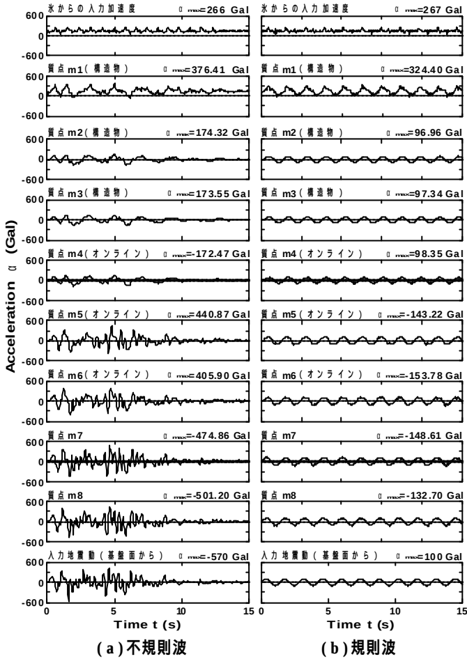
図-4 入力加速度と応答加速度の時刻歴
