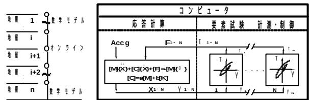
図-1 オンライン動的応答実験の概念図
