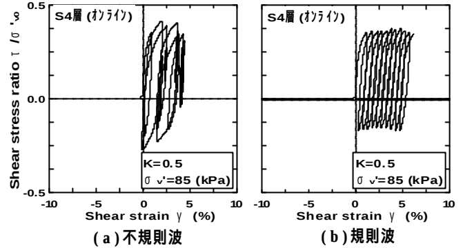
図-5 せん断応力比 - せん断ひずみ関係
