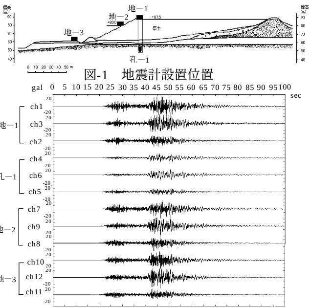
図-2 加速度波形記録
