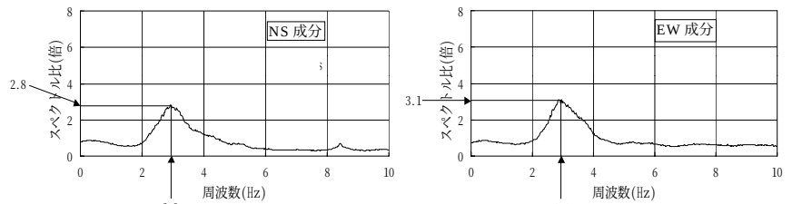
図-4 常時微動の増幅率
