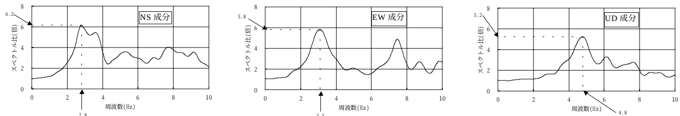
図-3 地震動の増幅率
