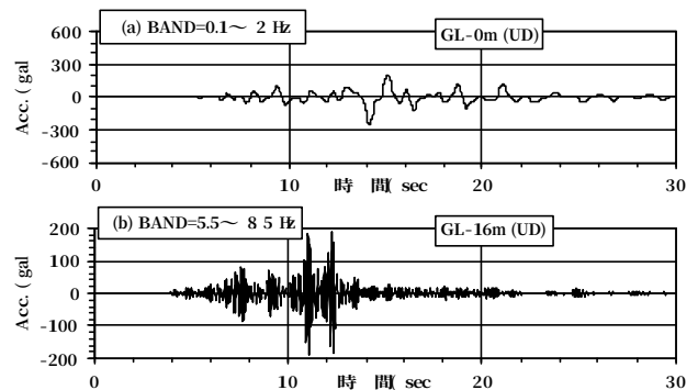
図-4 バンドパス・フィルタ通過後の波形
