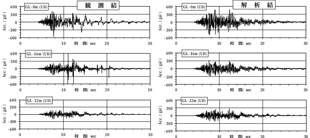
図-2 加速度時刻歴における観測結果と解析結果の比較
