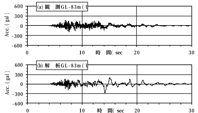
図-5 地表面波形を入力した場合の解析
