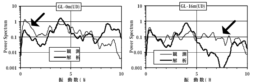
図-3 パワースペクトルの比較
