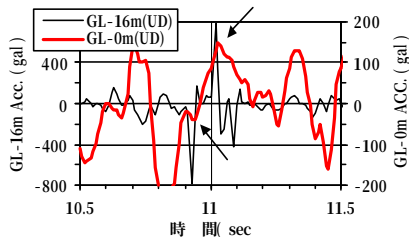
図-7 パルス波の位相 (2)
