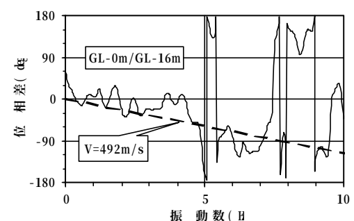
図-1 GL-0m/-16m 間のフェイズスペクトル
