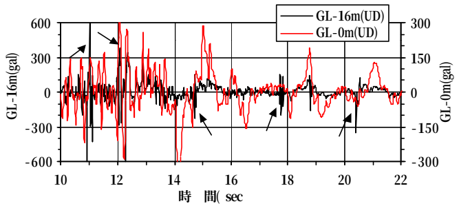
図-6 パルス波の位相 (1)
