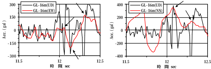
図-8 UD成分と水平動の対応
