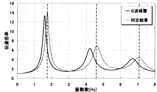
図-4 S波検層と同定速度構造の伝達関数 (縦の破線は弱震動地震記録の固有振動数を示す)
