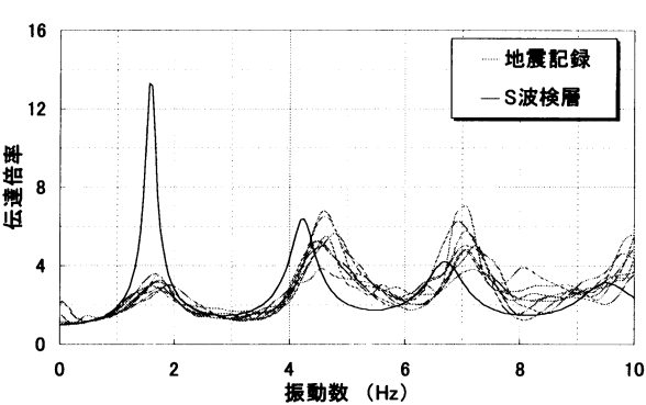
図-2 S波検層結果および弱震動地震記録の伝達関数
