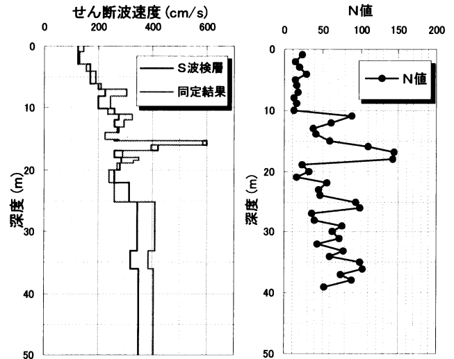
図-3.1 S波速度構造の比較
