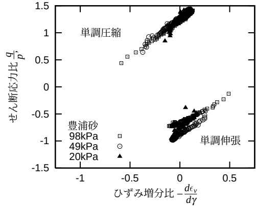
図4 豊浦砂の応力-ダイレイタンシー関係
