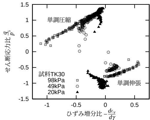
図5 試料 TK30 の応力-ダイレイタンシー関係
