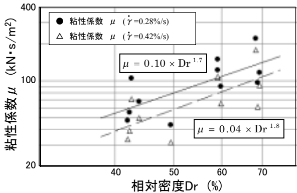
図 2 粘性係数と相対密度の関係(中空ねじり試験)
