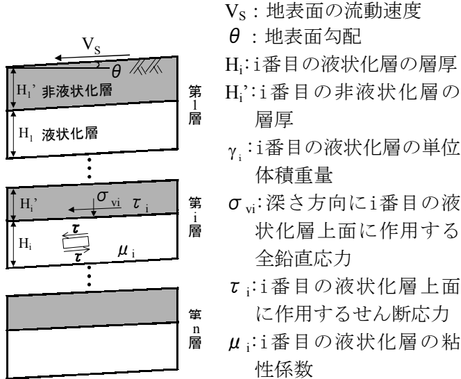
図5 傾斜地盤の液状化層の流れ
