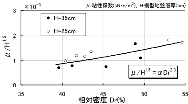
図 1 粘性係数と相対密度の関係(重力場の流動実験)
