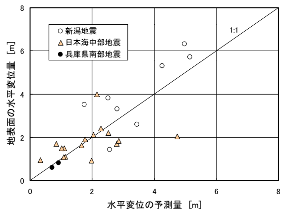
図6 式(8)による予測値と実測地表面水平変位量の関係
