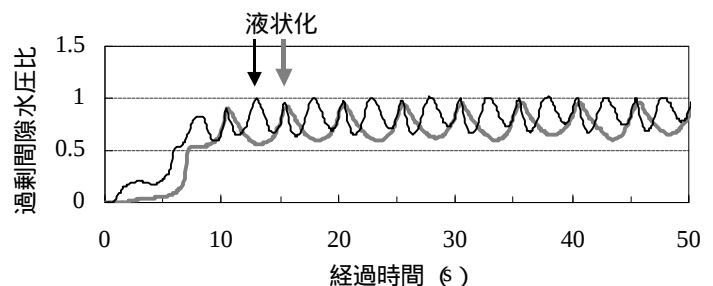
図 - 3 過剰間隙水圧比の時刻歴
