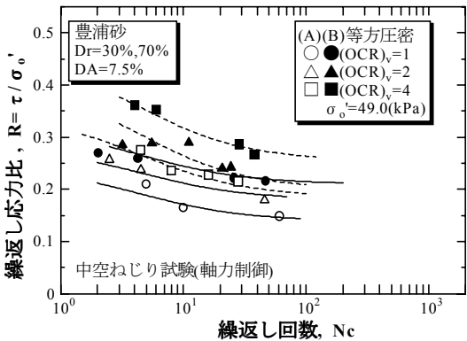
図 1 繰返し応力比と繰返し回数の関係 ( R = \tau / \sigma'_0 )
