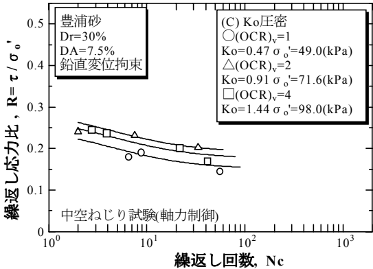
図 2 繰返し応力比と繰返し回数の関係 ( R = \tau / \sigma'_0 )
