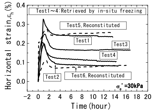
図5 江戸川砂の融解時の水平ひずみ
