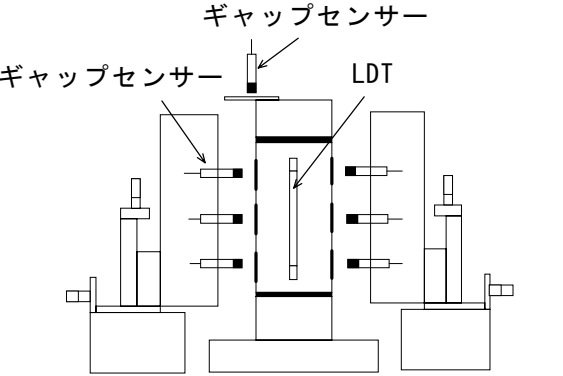
図3 供試体融解時のひずみ測定装置装置
