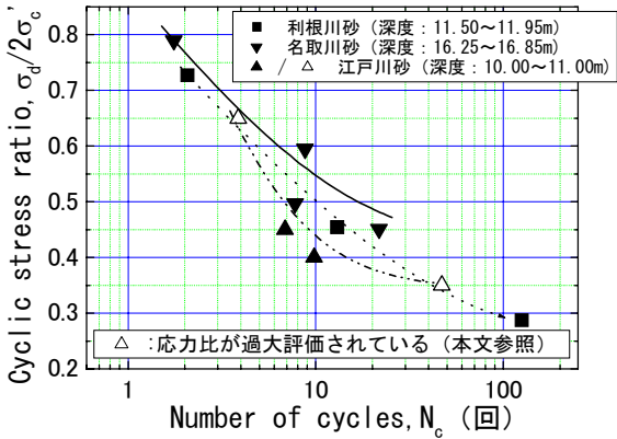
図1 各試料の液状化強度曲線
