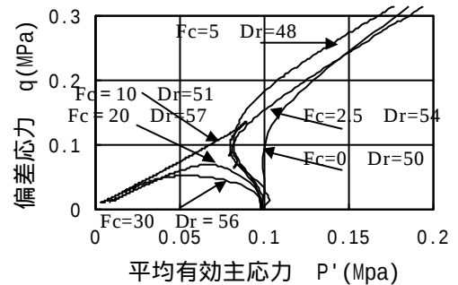
図-5 有効応力経路図
