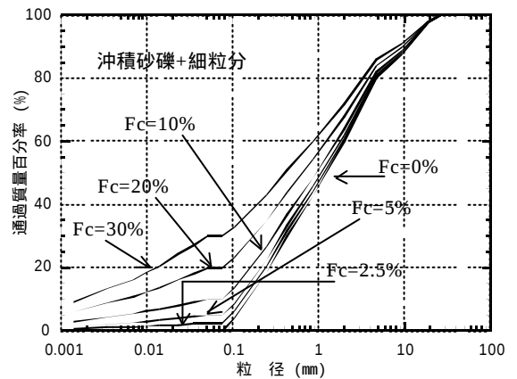
図-2 粒度分布
