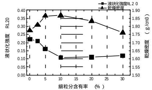
図-4 液状化強度と細粒分含有率の関係
