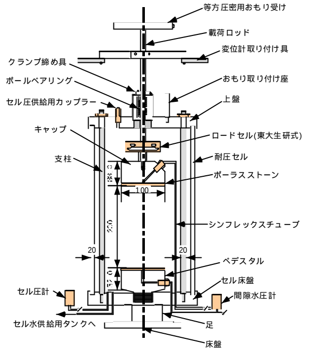
図-1 三軸圧縮試験機
