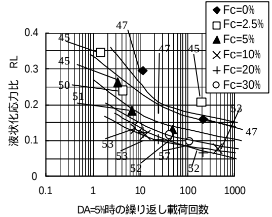
図-3 Dr 50%の液状化強度曲線
