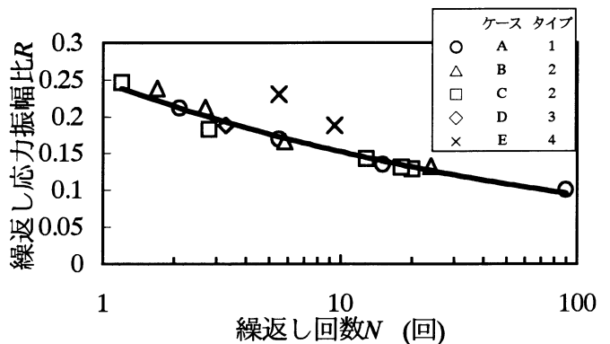
図-4 液状化強度曲線
