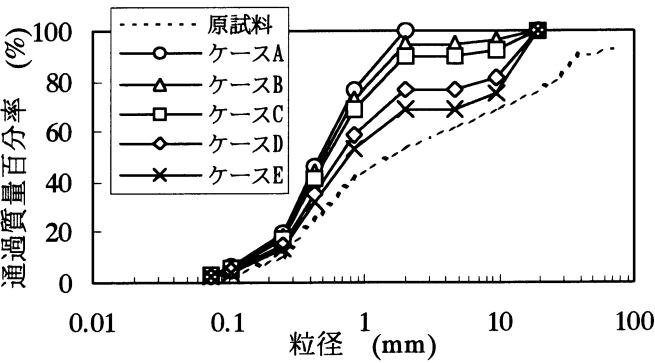
図-2 原試料および各ケースの粒径加積曲線
