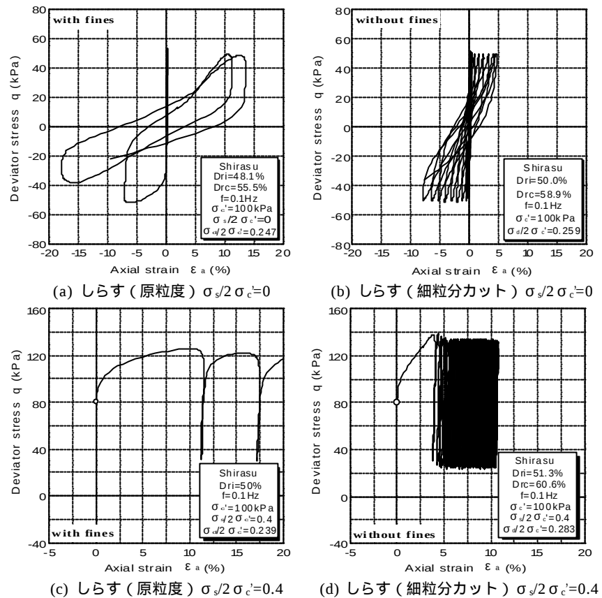
図-3 軸差応力 - 軸ひずみ関係
