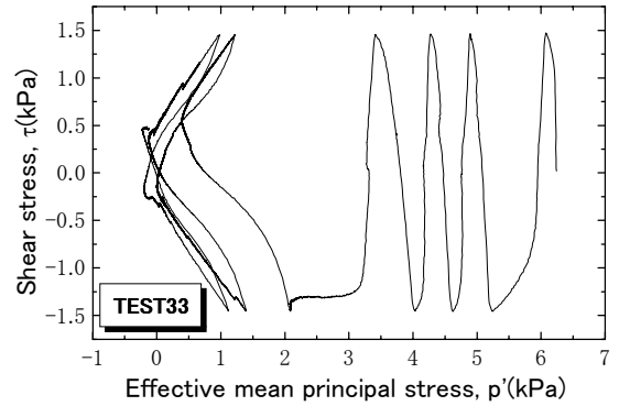
図3 ケース4の有効応力経路の例
