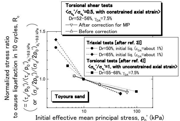
図5 液状化強度に及ぼす拘束圧の影響
