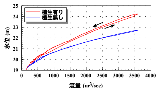
図-6 水位-流量曲線
