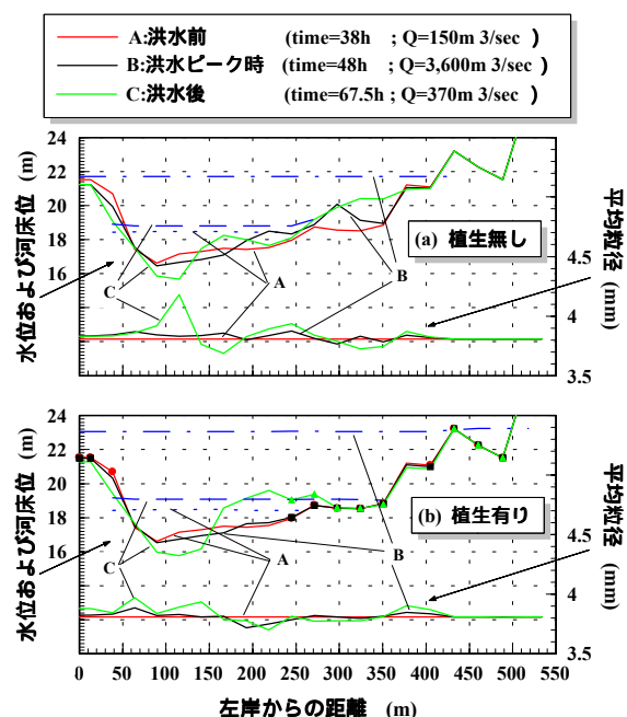
図-3 河床横断形状および河床材料の平均粒径
