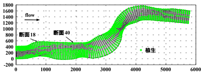
図-2 計算対象領域および植生分布
