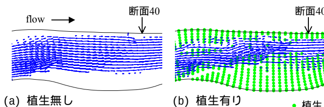
図-5 植生の有無による流況の比較 (Time=45hr)
