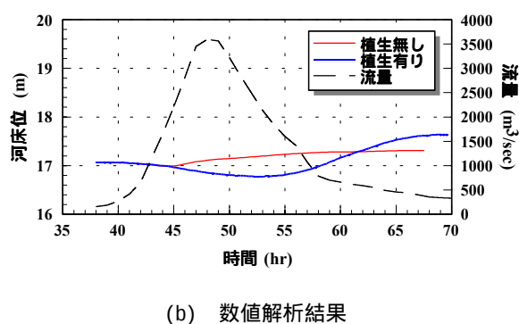
図-4 現地調査と数値解析による河床変動の比較
