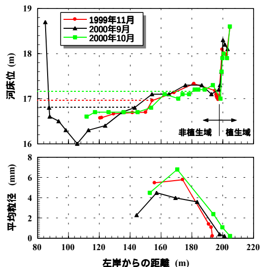
図-1 河床位および河床材料の平均粒径
