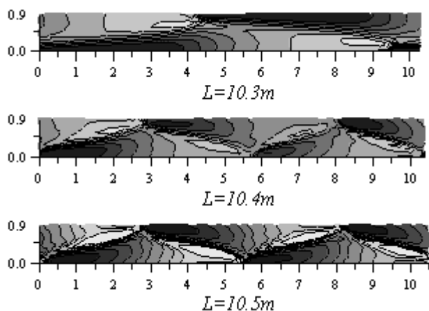
図-3 河床コンター図
