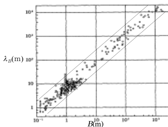
図-5 川幅と波長の関係
