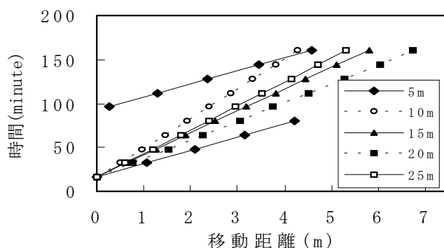
図-1 砂州前縁の走時曲線
