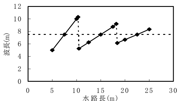
図-2 砂州波長と水路長の関係
