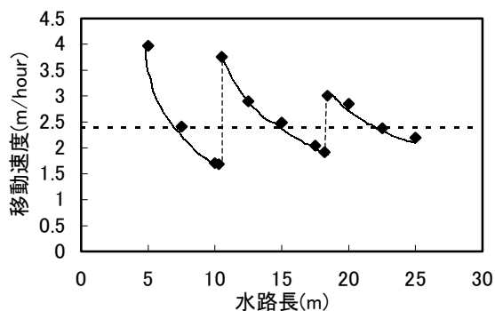
図-4 砂州の移動速度と水路長の関係
