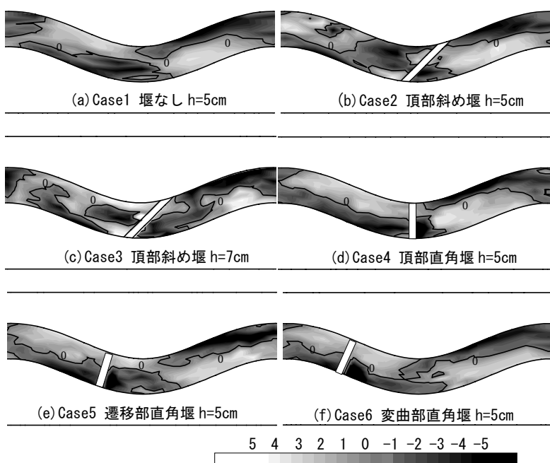
図-4 河床変動コンター
