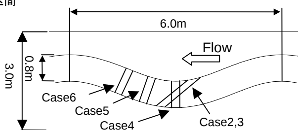
図 - 2 堰設置位置
