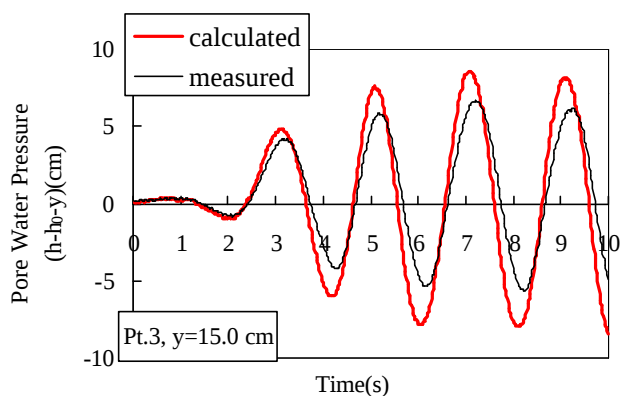
図4 実験値と解析値（空気含有率0.5%）の比較
