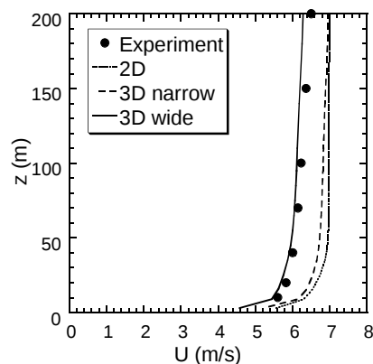
図2 C点での平均風速の鉛直分布（北東風）
