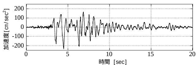
(a) X方向に入力した地震動
