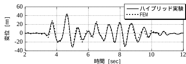
(b) 変位応答
