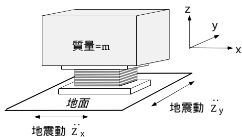
図-1 ハイブリッド実験で想定した構造系
