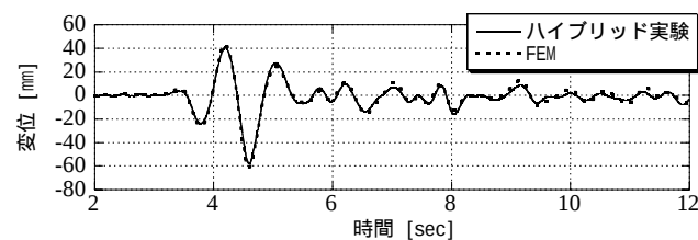
(d) Y方向の変位応答
