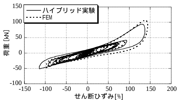
(e) X方向の復元力特性
