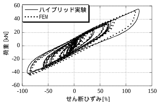
(c) 復元力特性の比較
