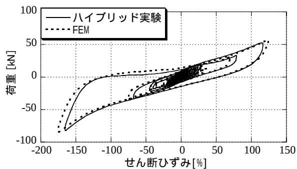
(f) Y方向の復元力特性
