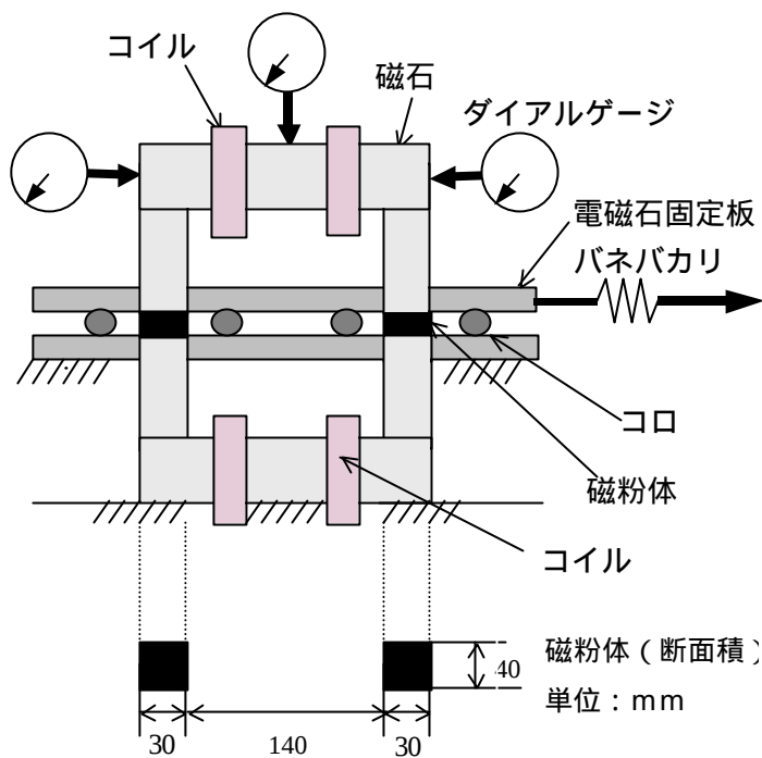
図-1 実験装置
