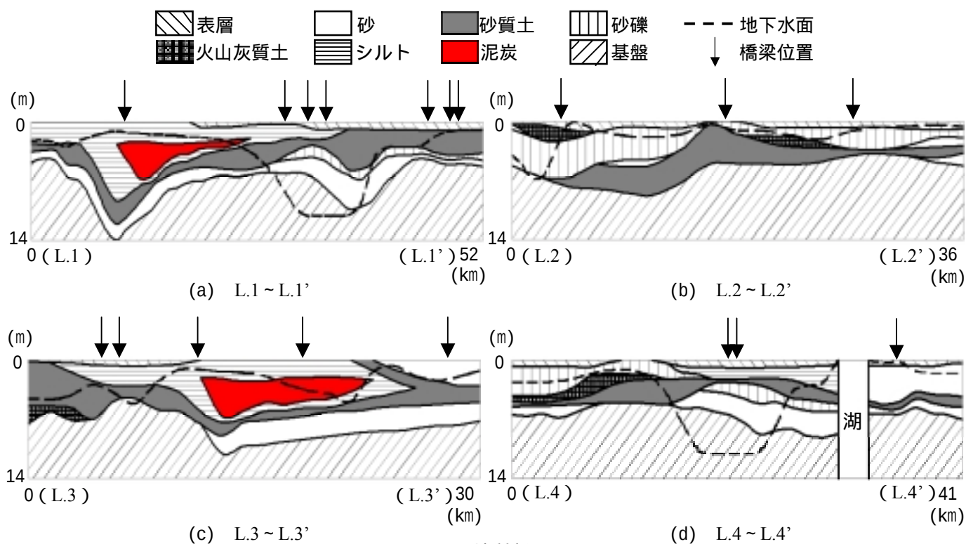
図 - 2 地質断面図
