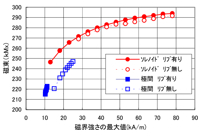
図2 新旧磁化器の磁化特性の差
