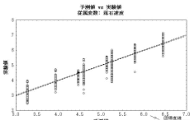
図 2 (a) 30・40 度 予測値と実験値の散布図 落石形状を含まない場合
