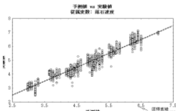
図 2 (b) 30・40 度 予測値と実験値の散布図 落石形状を含む場合
