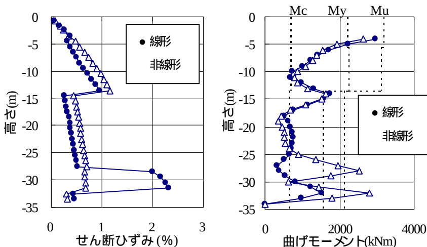
図-3 自由地盤系の最大せん断ひずみ分布
