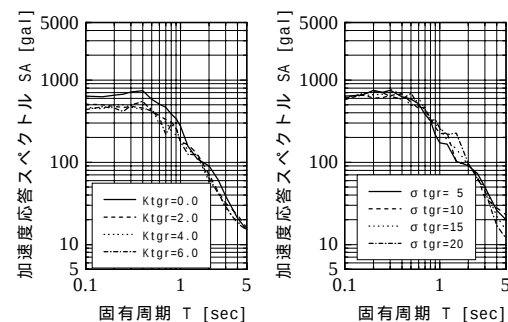
図-3 加速度応答スペクトル(タイプ II, I 種地盤, \mu=4 )
