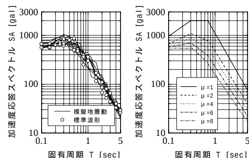
図-4 加速度応答スペクトル ( \mu=4 )
