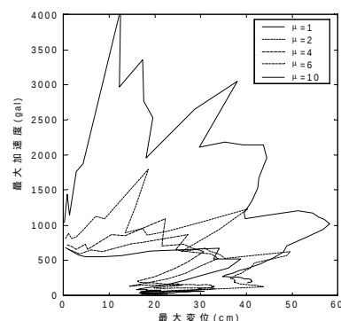
図 3 必要変位-強度スペクトル
