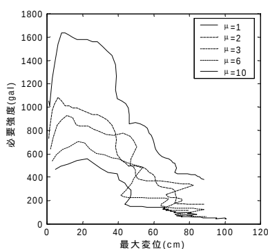
図6 必要変位-強度スペクトル(JR)
