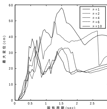
図 2 変位応答スペクトル
