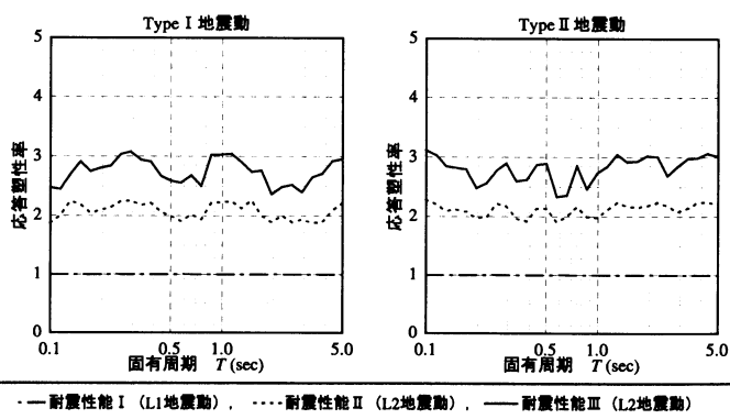
図-3 損傷度指標の限界値を満たす必要塑性率スペクトル (許容塑性率 \mu=3 )
