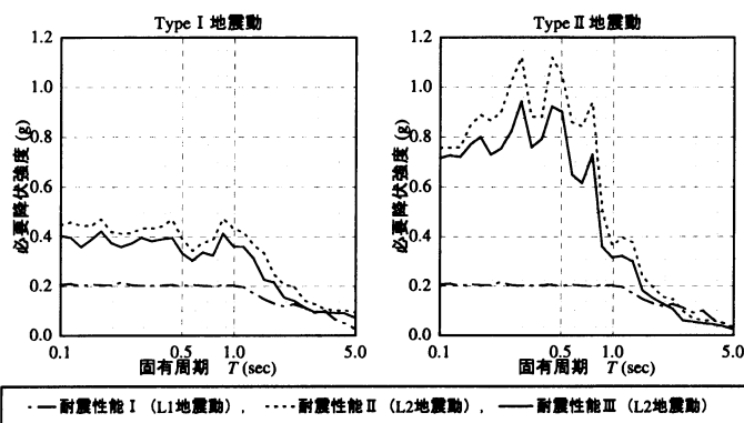
図-2 損傷度指標の限界値を満たす必要降伏強度スペクトル (許容塑性率 \mu=3 )
