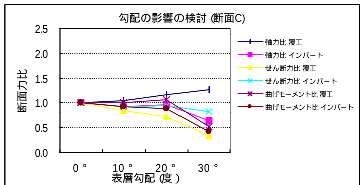
図4：断面力比(ケースC)
