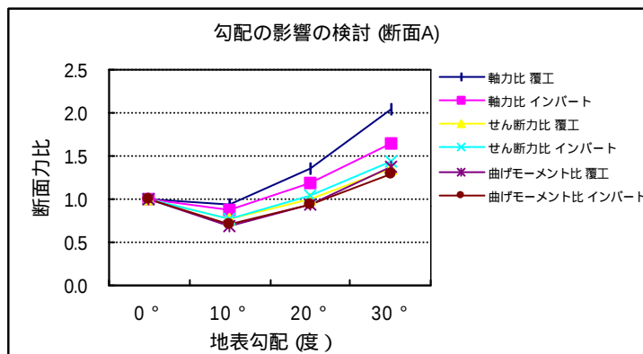
図2：断面力比（ケースA）
