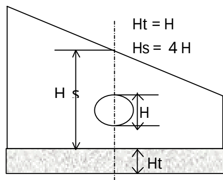
図 1 傾斜地盤での代表深さ H_s の取り方
