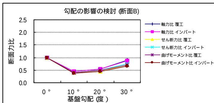
図3：断面力比（ケースB）
