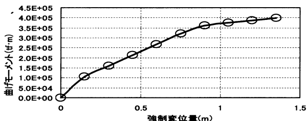
図-10 縦ずれ断層の最大曲げモーメント
