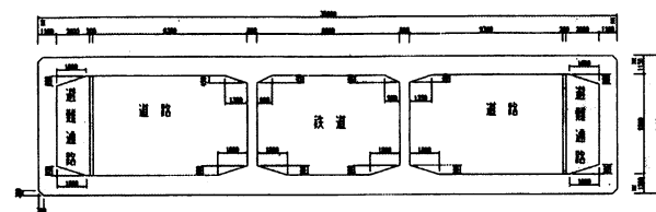
図-3 標準横断面図
