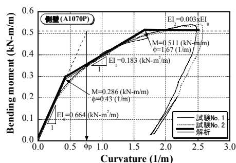
図-3 曲げモーメント-曲率関係の設定
