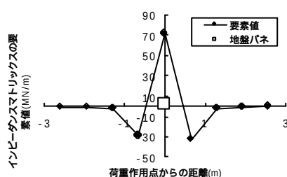
図-4 イビ°-ダ°要素値-着目点距離
