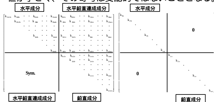
図-1 インピーダンス概念
