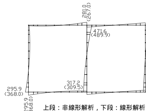
図 - 6 暗渠型曲げモーメントの比較(ケース 4)
