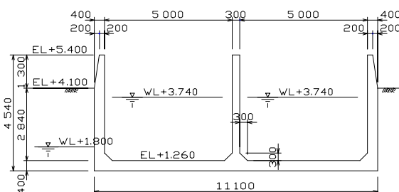
図-1 開渠型形状寸法
