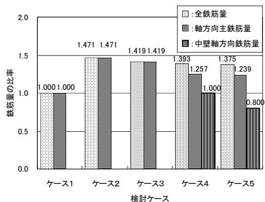
図 - 3 開渠型の鉄筋量の比率
