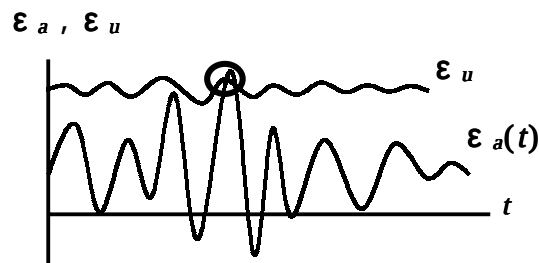
図1 動的解析に対する照査方のイメージ図
