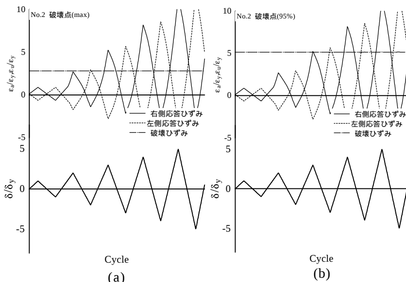
図2 応答ひずみ-最上端変位関係
