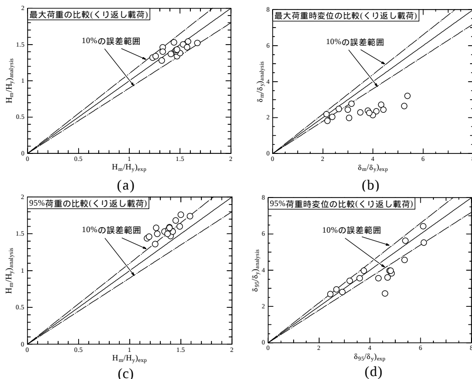
図3 実験値と解析値の比較
