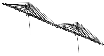
図-4 振動モード図(免震)
