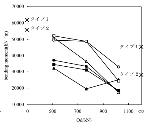
図-9 主塔基部の曲げ
