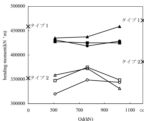
図-8 橋脚基部の曲げ
