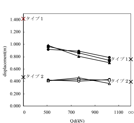
図-5 桁の最大変位
