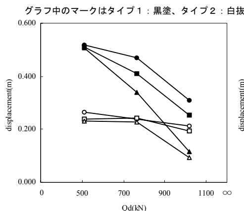
図-6 支承の最大変位
