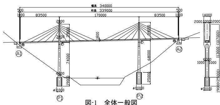
図-1 全体一般図
