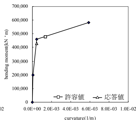
図-11 橋脚基部のM- \phi 関係 (免震)
