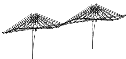
図-3 振動モード図(ピン結合)
