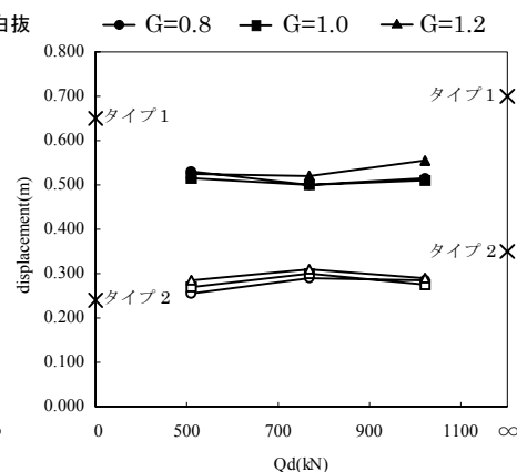
図-7 橋脚天端の最大変位
