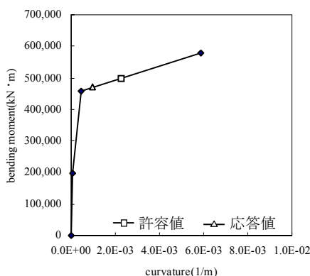
図-10 橋脚基部のM- \phi 関係 (ピン)
