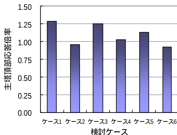
図-4 免震ケースによる塔頂変位比較
