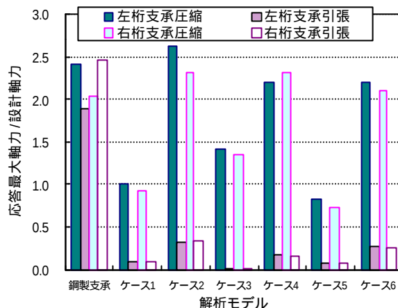
図-3 免震ケースによる応答軸力比較
