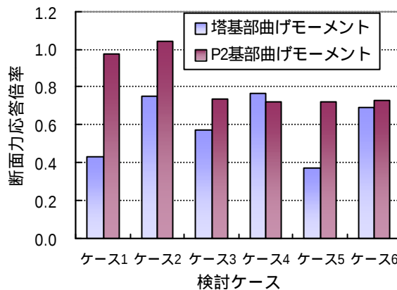
図-5 免震ケースによる応答断面力比較
