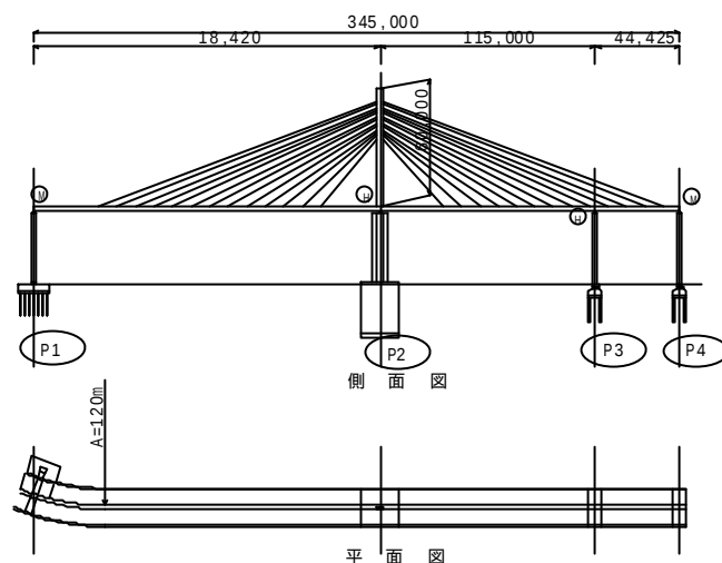
図-1 対象橋梁概略図
