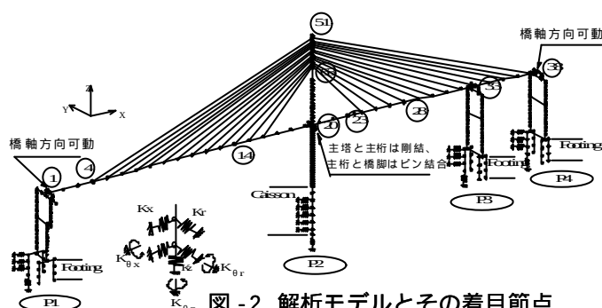
図-2 解析モデルとその着目節点
