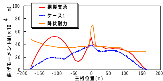
図-6 主桁面外応答曲げモーメント
