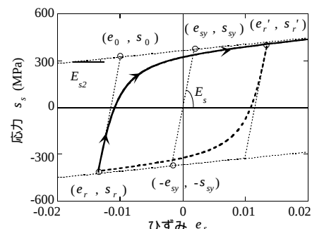
図4 Menegotto-Pinto モデル
