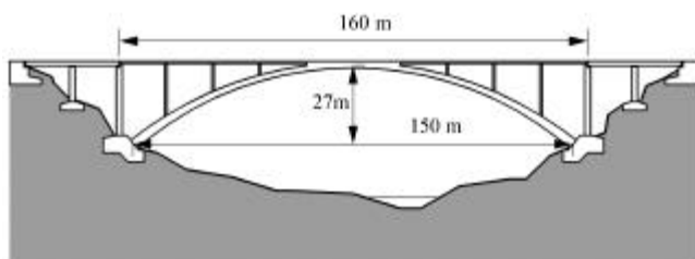
図1 解析対象とする RC アーチ橋
