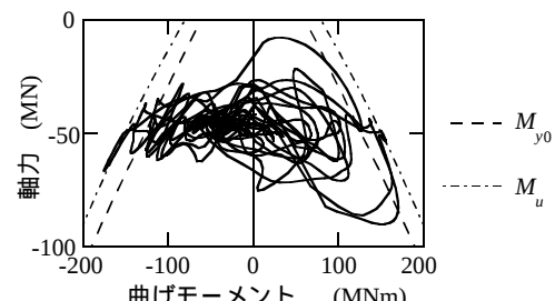
(b) 軸力～曲げモーメントの履歴
