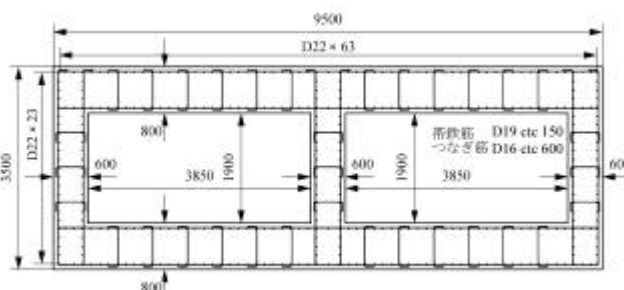
図2 スプリング部の配筋
