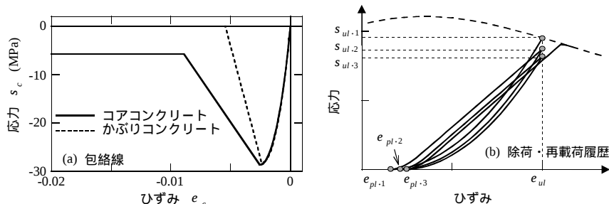
図3 コンクリートの応力度～ひずみモデル
