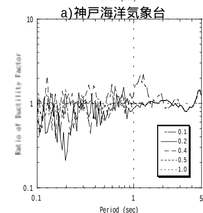
図-2 降伏震度による塑性率の比率
