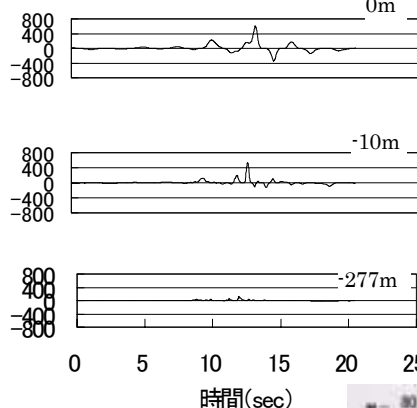
図-7 エネルギー波形
