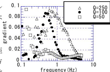
図-9 距離増加係数 (異方多重散乱モデル, \mu=2 , 内部減衰あり)
