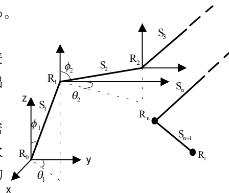
図-1 n次散乱のモデル
