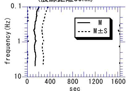
図-3 平均・分散群遅延時間 スペクトル
