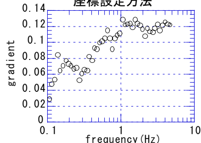
図-8 距離増加係数 (異方多重散乱モデル, \mu=4 )
