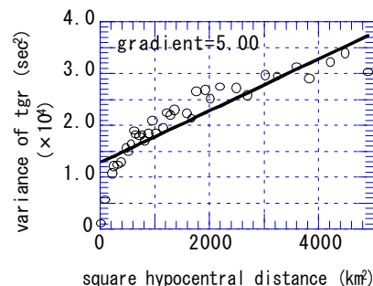
図-4 分散群遅延時間スペクトルの 距離増加の様子
