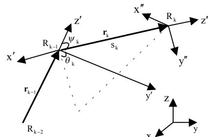
図-7 異方多重散乱モデルの 座標設定方法
