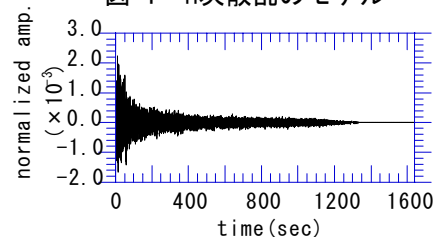
図-2 グリーン関数 (震源距離30km)
