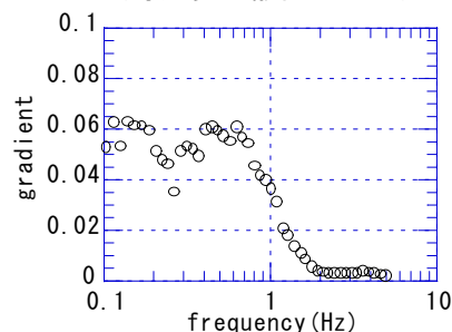
図-6 距離増加係数 (観測記録)
