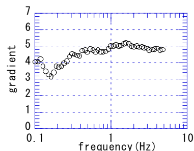
図-5 距離増加係数 (等方多重散乱モデル)
