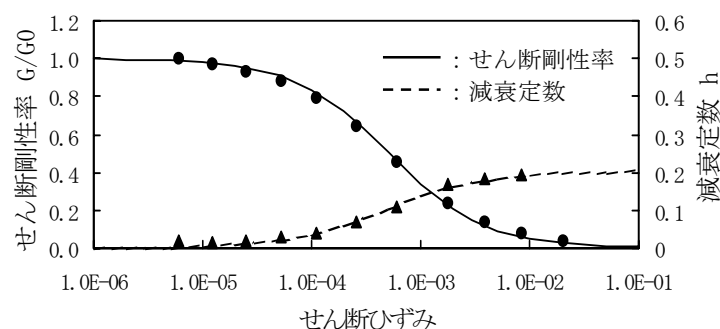
図-3 砂礫層（崖錐層）の動変形特性
