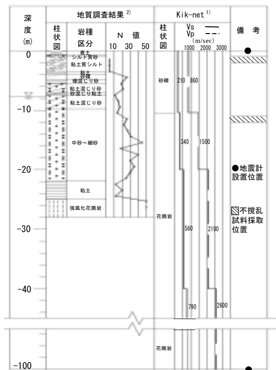
図-2 地盤概要
