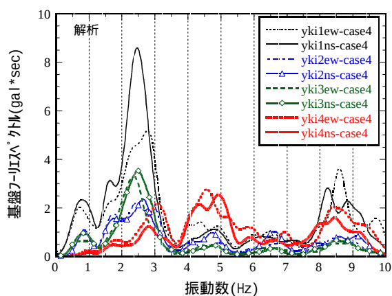
図-4 観測と解析の基盤フーリエスペクトル（四日市港）
