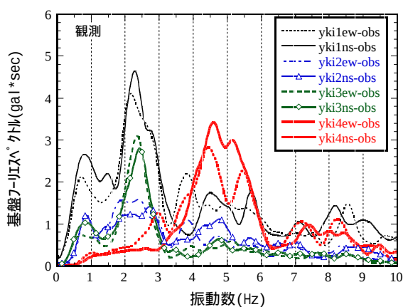
図-4 観測と解析の基盤フーリエスペクトル（四日市港）
