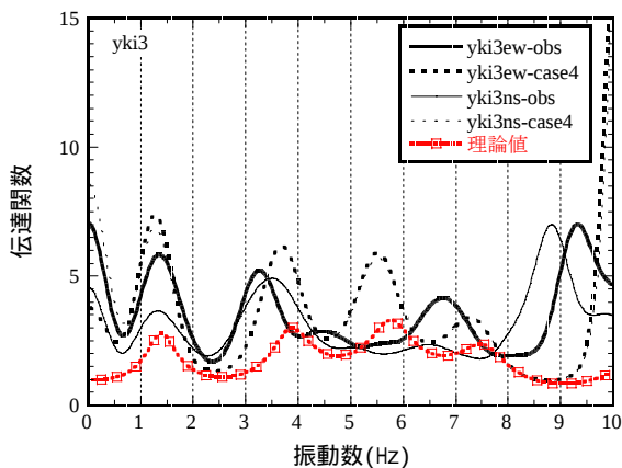
(1)加速度（小）
