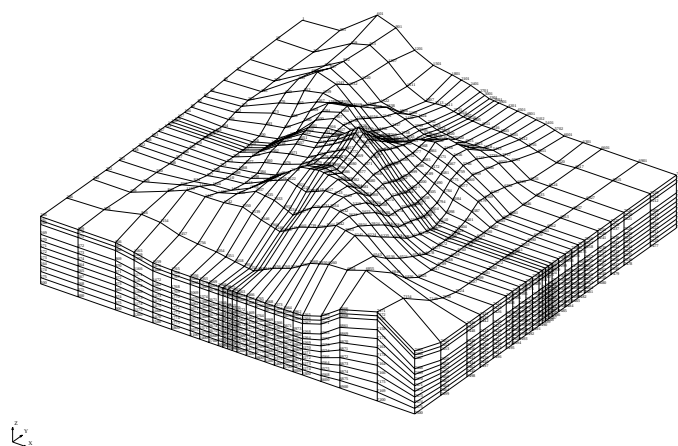
図-2 3次元解析モデル
