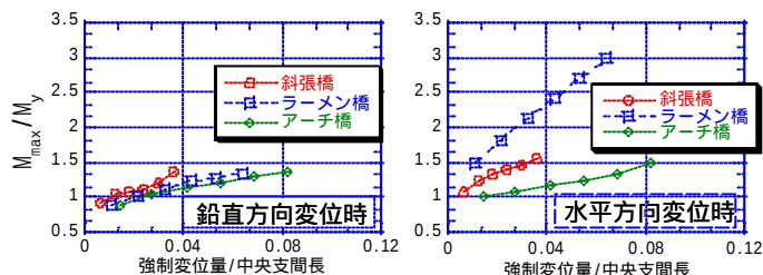
図-2 橋種の違いによる損傷進展度
