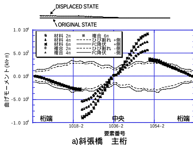
a) 斜張橋 主桁
