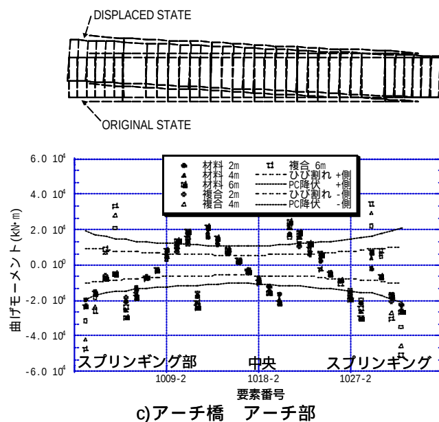
図-3 水平方向にそれぞれ2, 4, 6m変位させた場合における曲げモーメントの最大値分布
