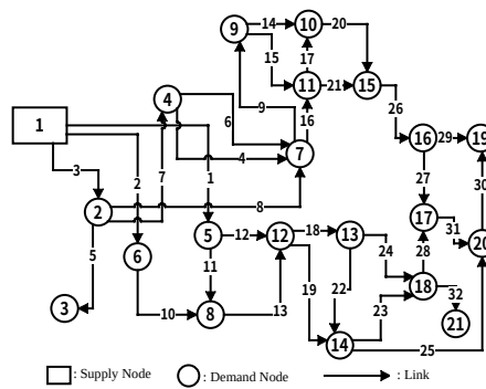
図-2 上水道システム
