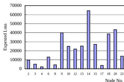
図-3 期待損失給水量
