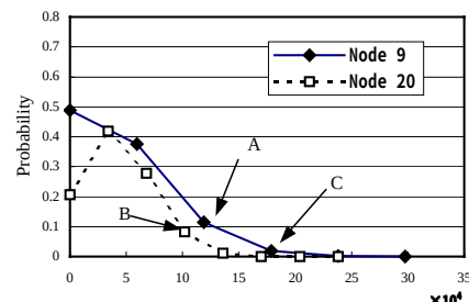
図-4 損失確率関数 1
