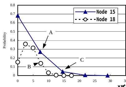
図-5 損失確率関数 2
