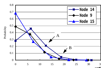
図-6 損失確率関数 3
