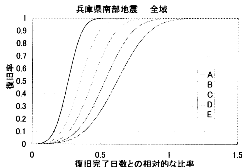
図6 地震動強度別復旧曲線 (ガス施設：兵庫県南部地震 全域)
