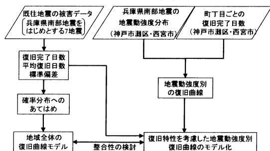
図1 地震動強度別復旧曲線のモデル化の方法
